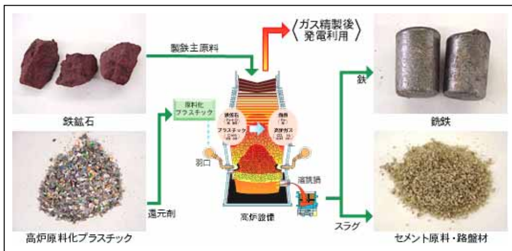
使用済みプラスチックの高炉原料化
